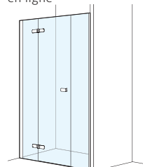
Porte pivotante avec paroi latérale en ligne
