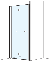
Porte pliante battante en 2 parties en niche
