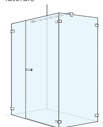
Porte battante avec paroi latérale en ligne charnières sur la paroi latérale
