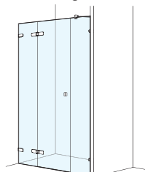
Porte pivotante avec élément fixe et paroi latérale en ligne en niche
