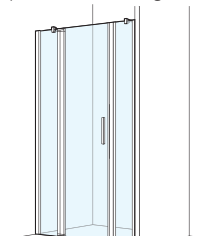
Porte battante avec élément fixe et paroi latérale en ligne
